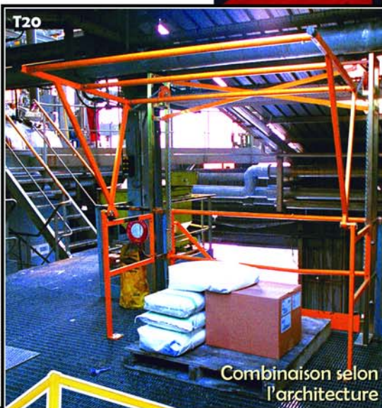
Reprise des charges au palan
